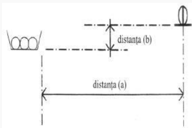
Figura 7.16 - Distanțe de amplasare a sprinklerelor față de obstacole care sunt în întregime sub nivelul deflectorului (a) distanța măsurată pe orizontală de la sprinkler la fața unei grinzi sau a unui obstacol (b) distanța maximă între deflectorului amplasat deasupra părții inferioare a unei grinzi și un alt obstacol
