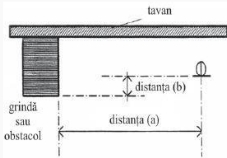
Figura 7.16 - Distanțe de amplasare a sprinklerelor față de obstacole care sunt în întregime sub nivelul deflectorului (a) distanța măsurată pe orizontală de la sprinkler la fața unei grinzi sau a unui obstacol (b) distanța maximă între deflectorului amplasat deasupra părții inferioare a unei grinzi și un alt obstacol
