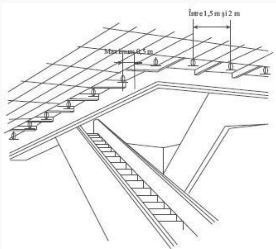
Figura 7.10 Amplasarea sprinklerelor în jurul golurilor din tavane
