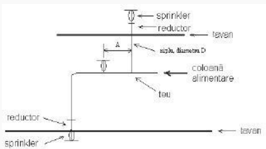
Figura 7.4. Amplasarea sprinklerelor în spațiul dintre nivelul tavanelor și a acoperișurilor
