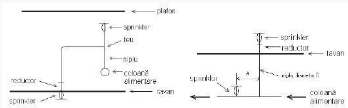
Figura 7.4. Amplasarea sprinklerelor în spațiul dintre nivelul tavanelor și a acoperișurilor
