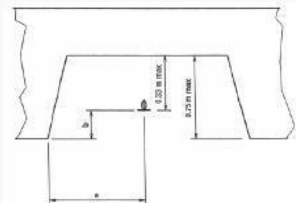
Figura 7.14 - Distanțe de amplasare a sprinklerelor față de marginea inferioară a unui plafon ondulat
